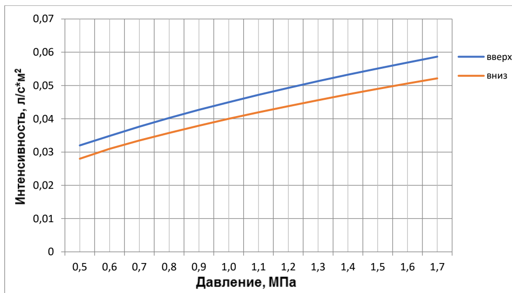
График зависимости интенсивности орошения от давления на площади 9 м2, защищаемой группой распылителей (два и более) с высоты 2,5 м
